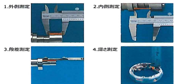
Ⅲ.ノギス 3-3. ノギスの測定使用例 (意外と多機能)
